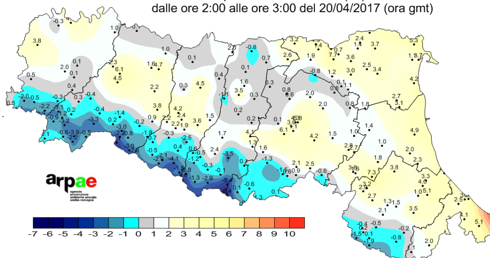
PUNTI - Temperatura media oraria (°C) dalle ore 2:00 alle ore 3:00 del 20/04/2017 (ora gmt)
